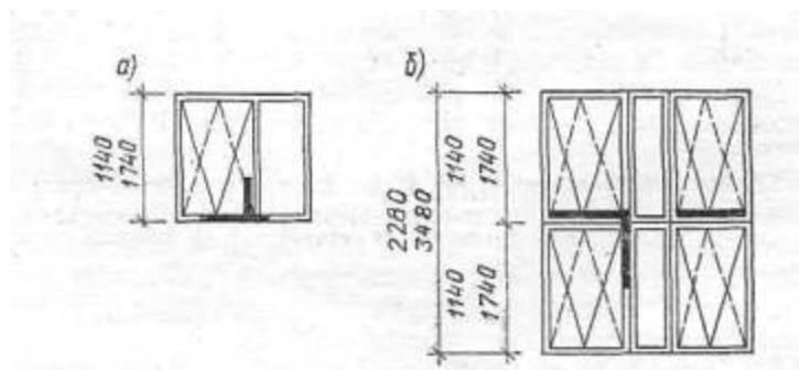
Рис. 1. Схемы установки и открывания фрамуг переплетов механизмами
