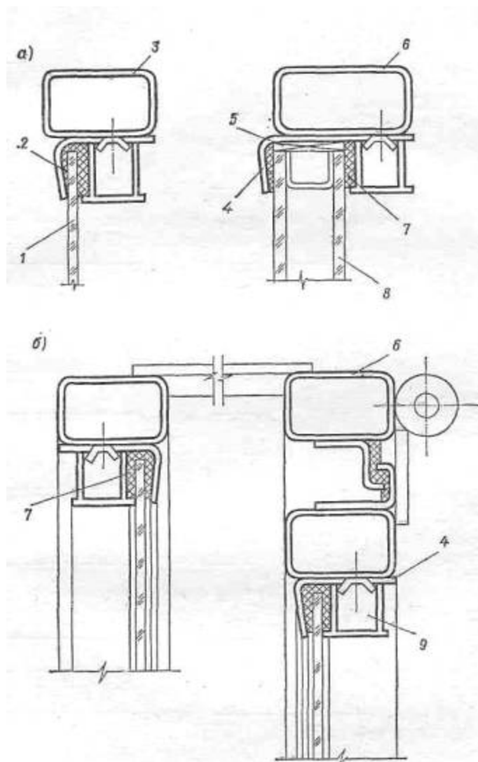
Рис. 3. Схемы сечений переплетов при остеклении
