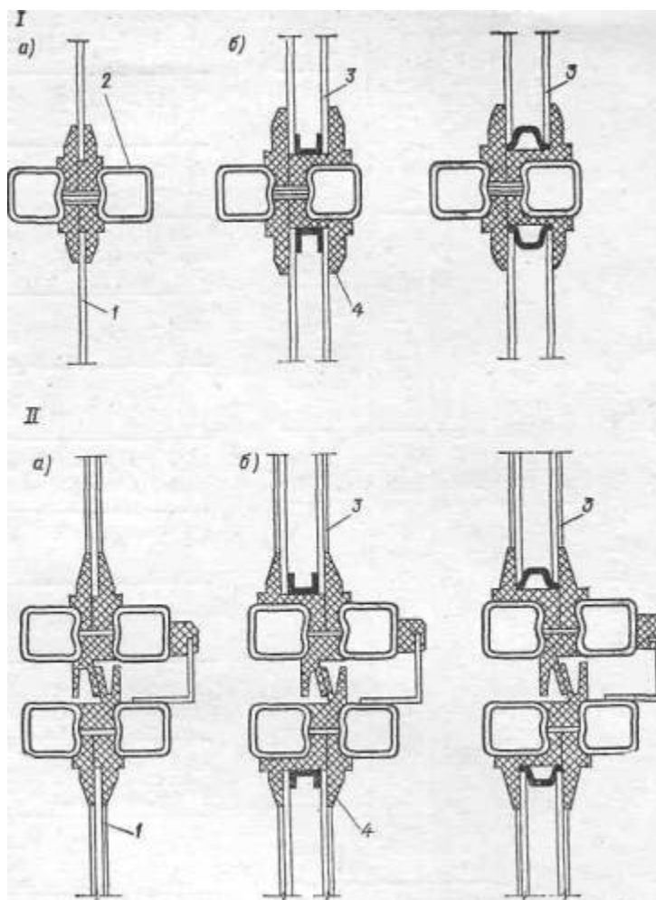
Рис. 2. Схемы сечений переплетов без фрамуг (I) и с фрамугами (II) при остеклении
