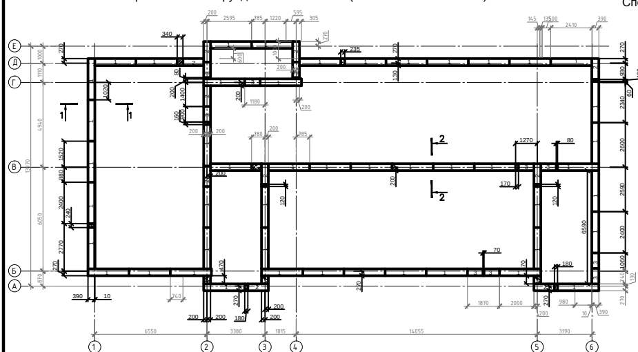
Схема расположения фундаментных блоков (низ на отметке +107.10)
