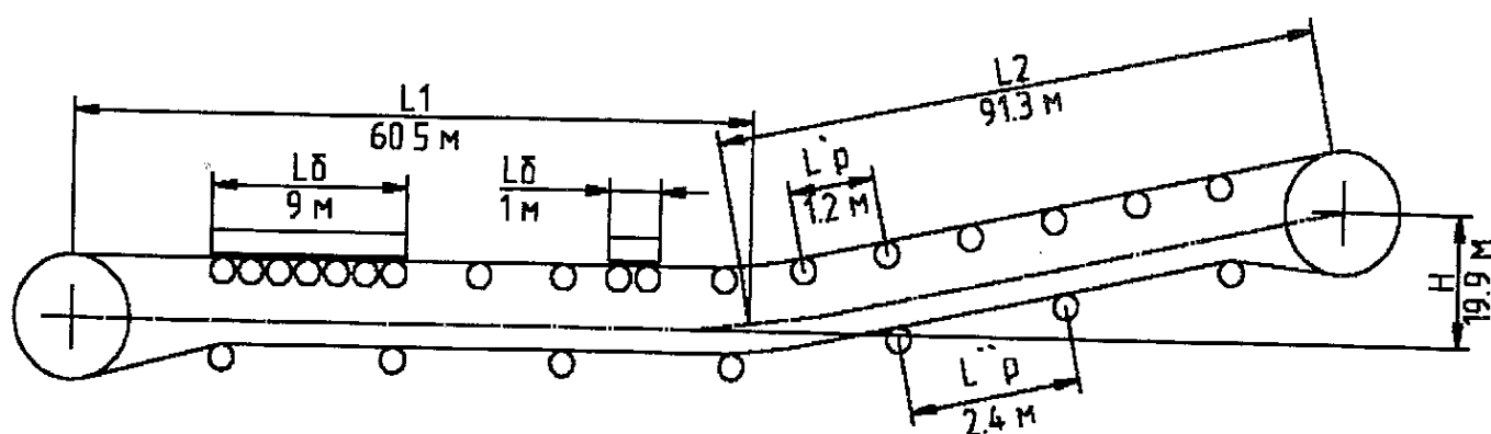
Рис. 1. Расчетная схема конвейера.
