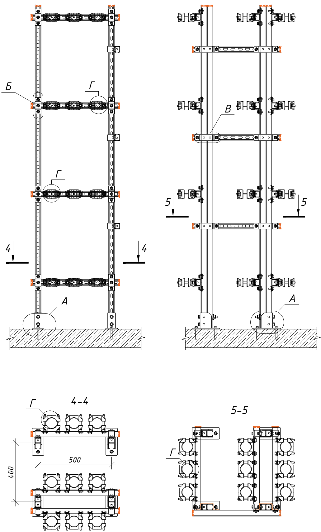
Рама для ВЗУ2, ВЗУ13, ВЗУ18
