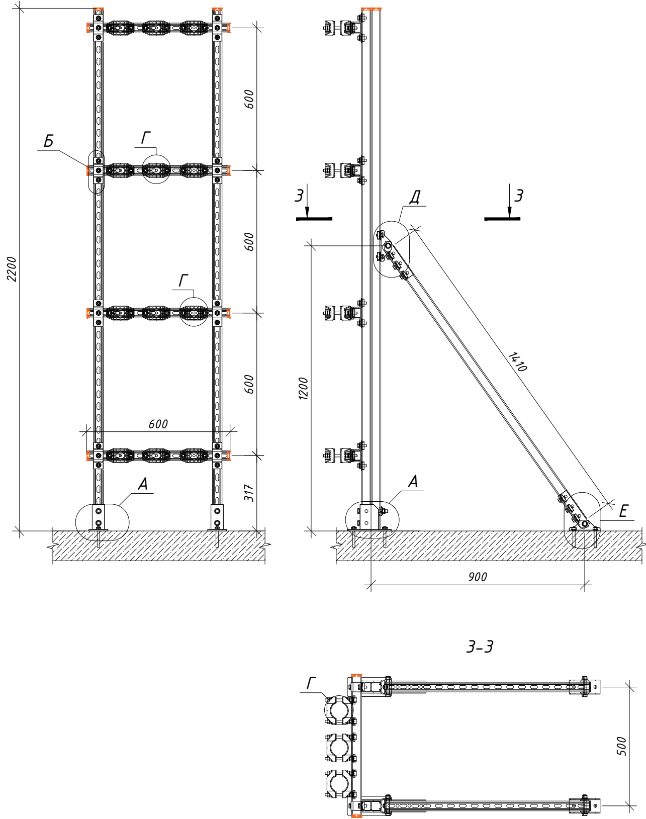
Рама для ВЗУ1, ВЗУ3, ВЗУ7, ВЗУ11, ВЗУ12, ВЗУ14, ВЗУ25, ВЗУ26
