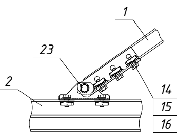
Узел Е
