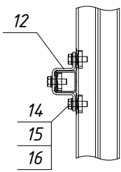
Узел Б
