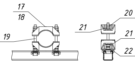
Узел Г
