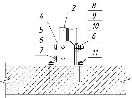
Узел Б
