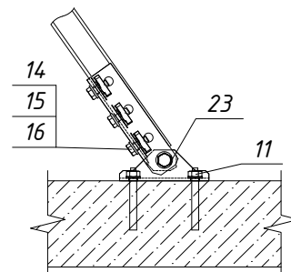
Узел Е
