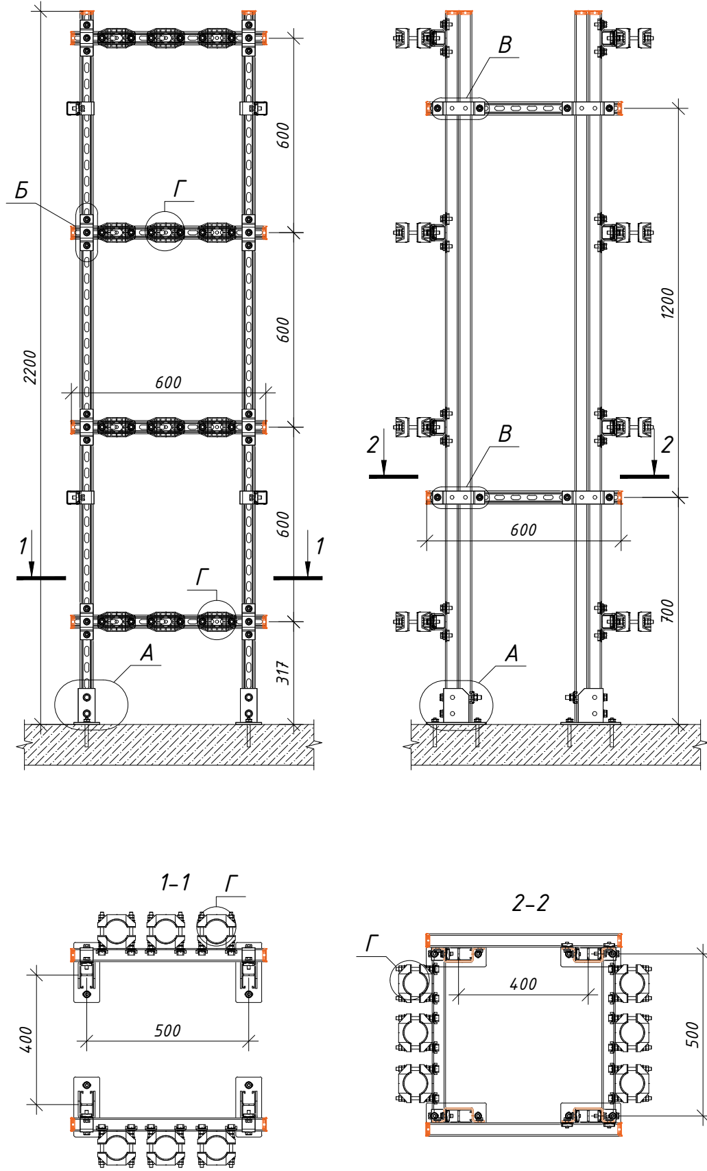
Рама для ВЗУ4, ВЗУ5, ВЗУ6, ВЗУ8, ВЗУ9, ВЗУ10, ВЗУ15, ВЗУ16, ВЗУ17, ВЗУ19, ВЗУ20, ВЗУ21, ВЗУ22, ВЗУ23, ВЗУ24
