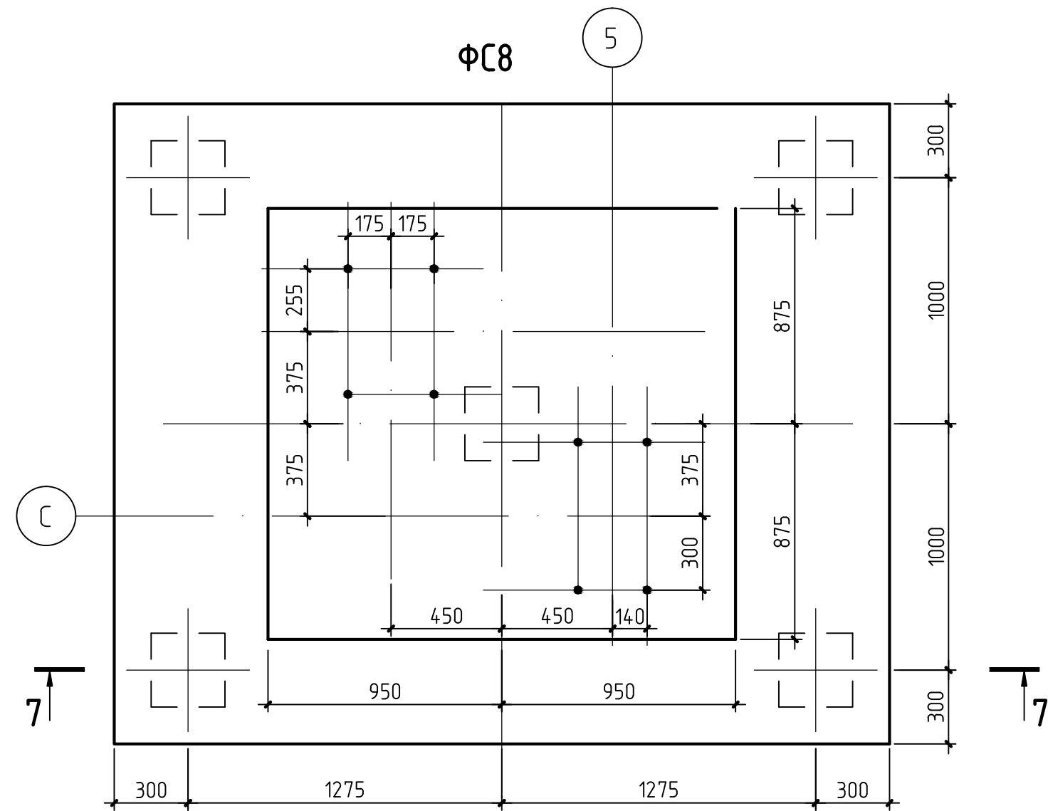
Схема армирования ФС8
