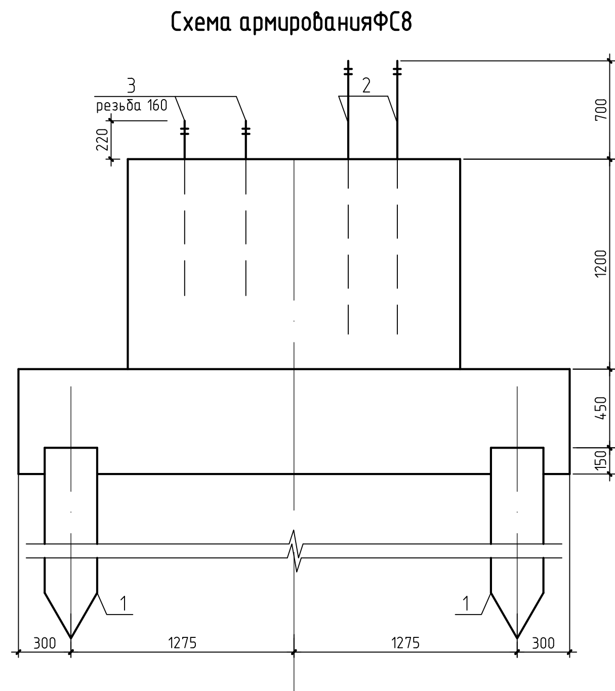
Схема армирования ФС8
