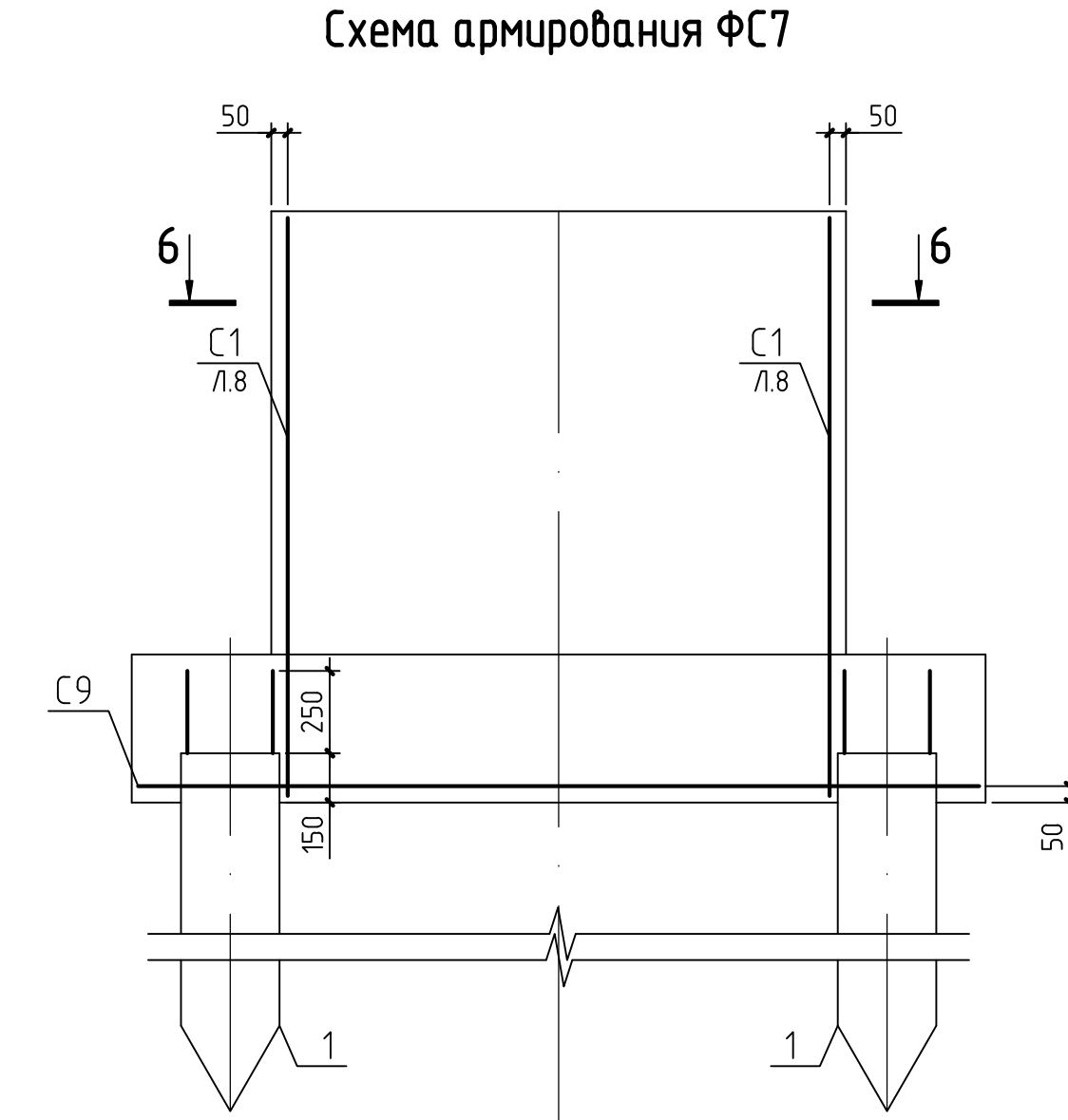
Схема армирования ФС7
