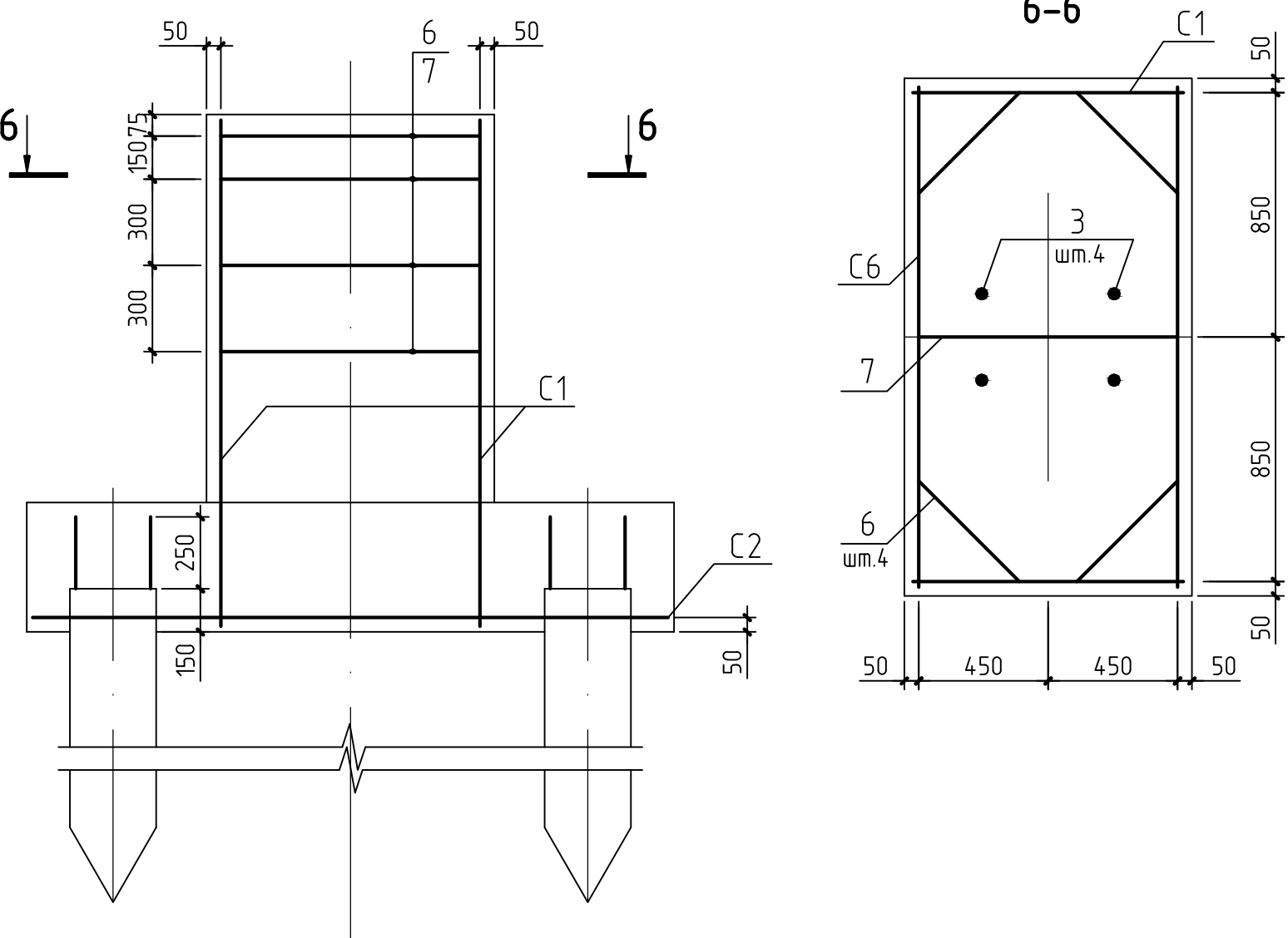
Схема армирования ФС4
