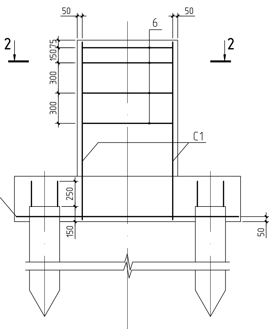
Схема армирования ФС1, ФС3
